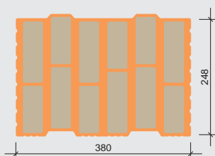
Przekrój pustaka Porotherm 38 T Profi
